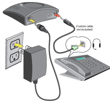
配合普通电话组合成电话会议终端
